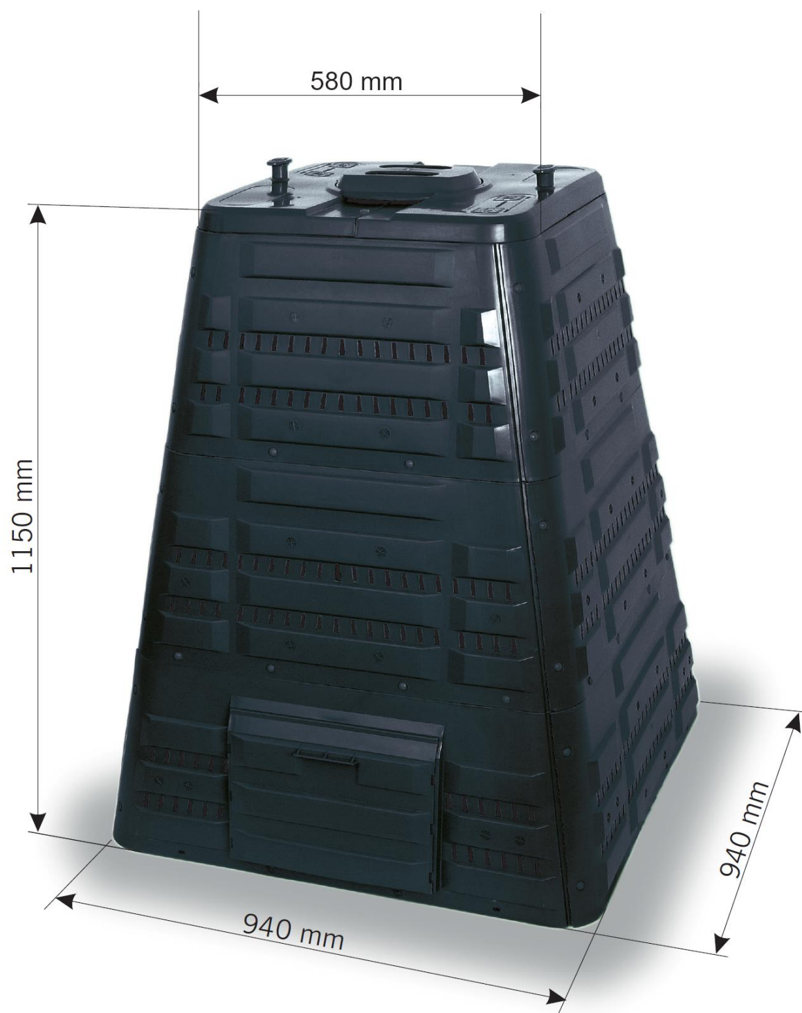
Rysunek techniczny z wymiarami Ekokompostownik TERMO-700 Czarny
